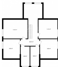
PASTOGĖ
