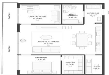
BUTO PLANAS 5 AUKŠTAS - 76,70 m 2
