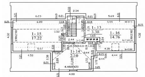
PASTOGĖS M1 PATALPŲ PLANAS
