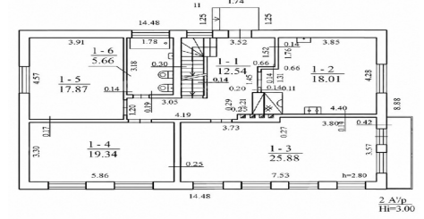
PIRMO AUKŠTO PLANAS
